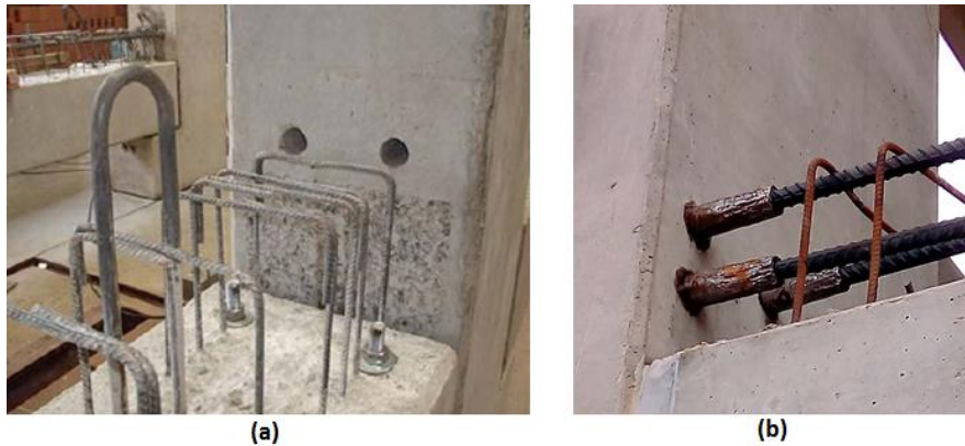
Figura 1 - (a) Ligação viga-pilar com furo para passagem de bainhas. (b) Ligação viga-pilar com uso de luvas.
